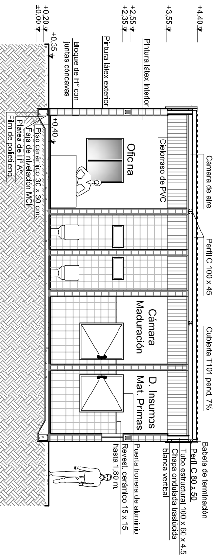
CORTE 1 - 1
